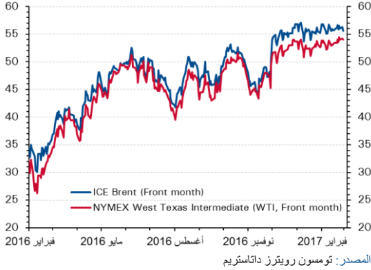
الرسم البياني ٢: منحنى أسعار العقود الآجلة لمزيج برنت (دولار للبرميل)
